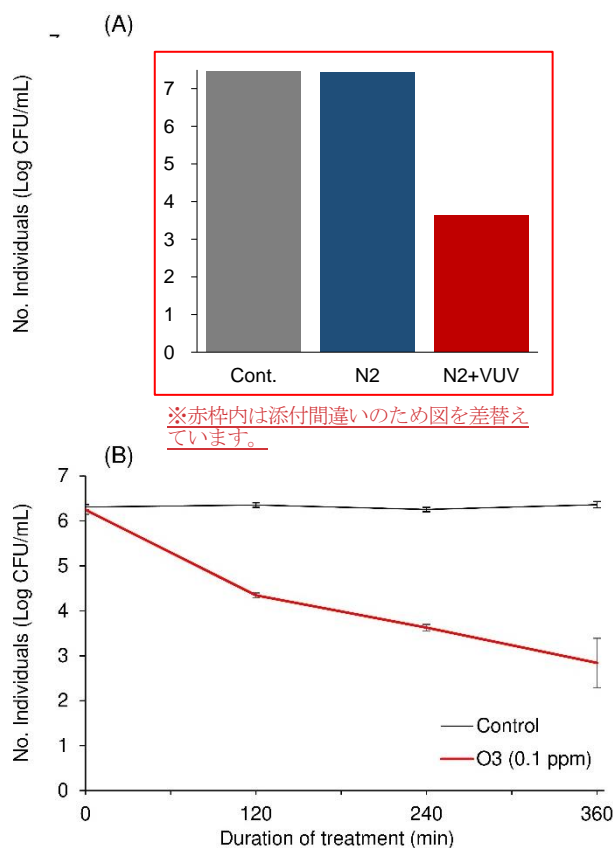
図 2. (A) VUV 照射または (B) 低濃度オゾン処理が大腸菌生菌数に及ぼす影響
